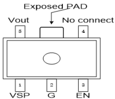
顶视图
